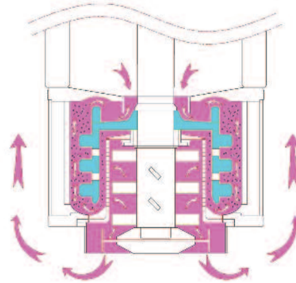
- 원료흐름도(내부) -
