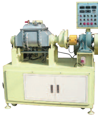
MODEL : U.K.25
