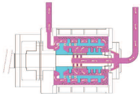
- 원료흐름도 -
